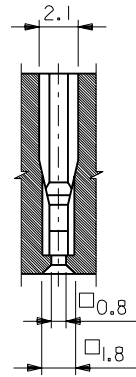
断面E-E SECT.E-E
